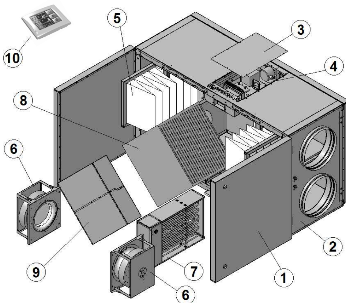
Состав установок
