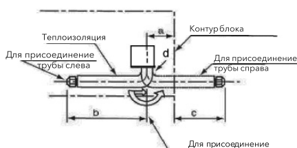
Труба газовой линии
