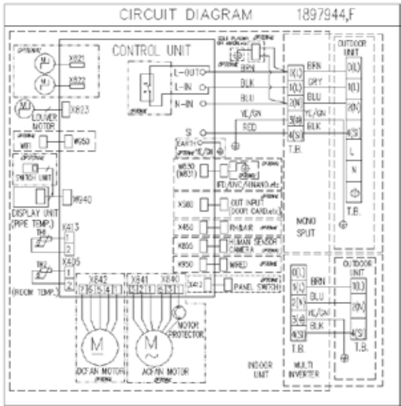
Внутренний блок KVAC-I-18IN-PT1, KVAC-I-24IN-PT1
