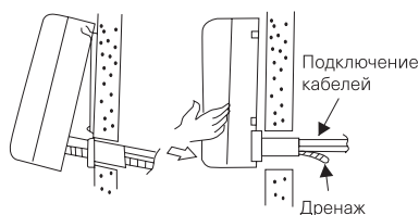
Монтаж дренажного трубопровода
