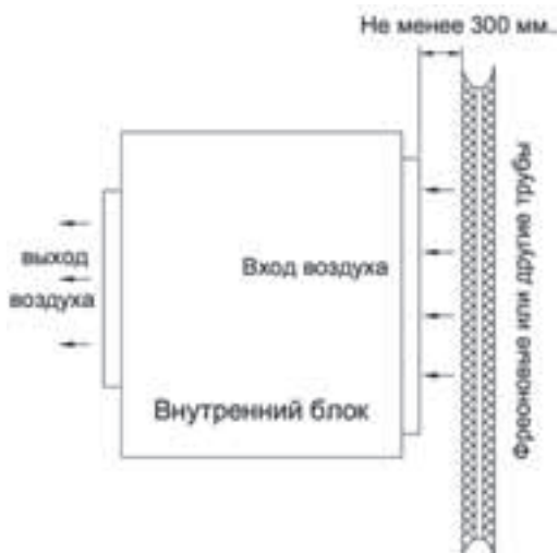
Рис. 6.5. Взаимное расположение фреоновых труб и внутреннего блока
