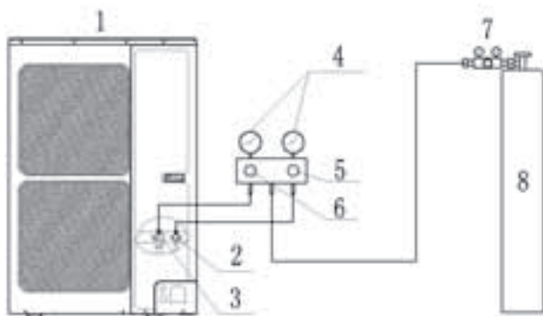
Рис. 6.14. Проверка на герметичность
