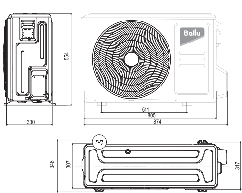
Размеры внешних блоков BM2OI-FM/out-14HN8_V1/EU, BM2OI-FM/out-18HN8_V1/EU:
