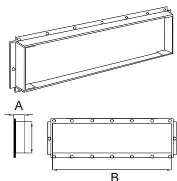
Фланец выхода воздуха
